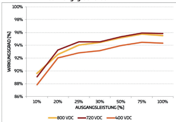
Wirkungsgradkurve
