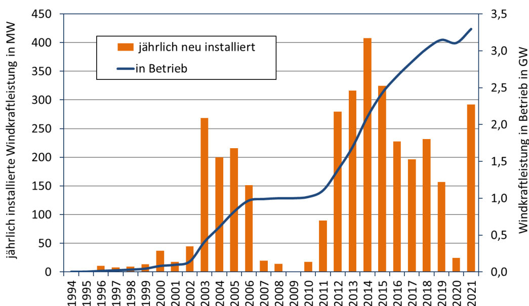
Abbildung 15 – Die Marktentwicklung der Windkraft in Österreich bis 2021 Quelle: IG Windkraft (2022)
