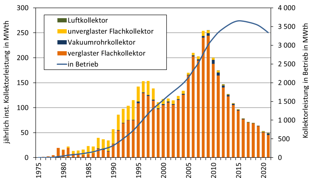
Abbildung 9 – Marktentwicklung der Solarthermie in Österreich bis 2021 Quelle: AEE INTEC (2022)
