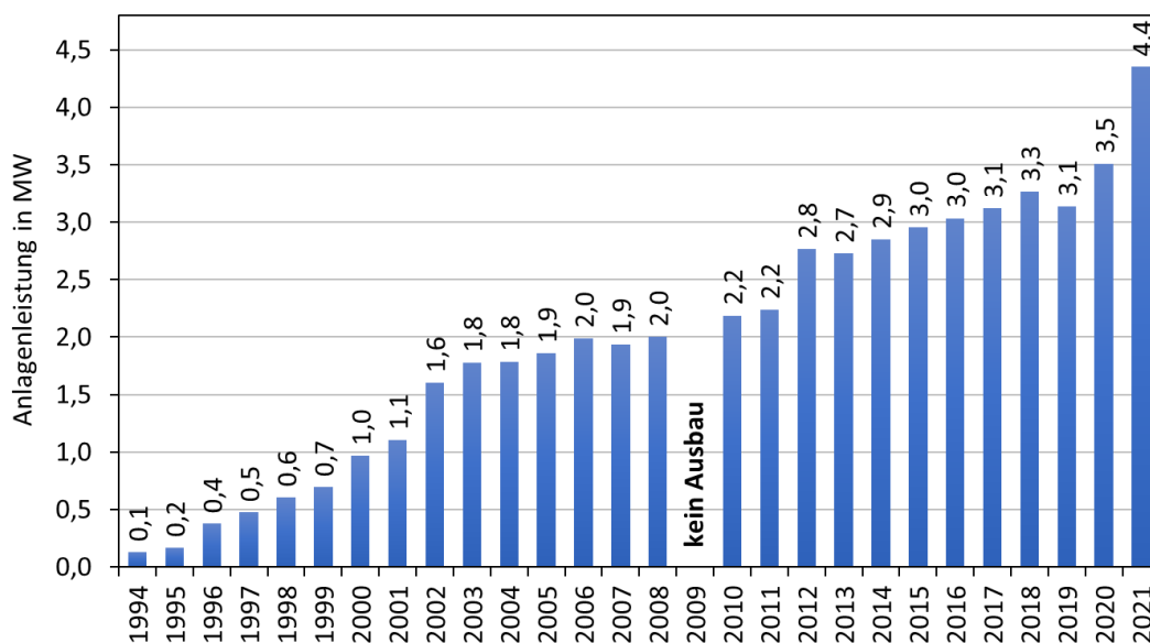
Abbildung 16 – Durchschnittliche Anlagenleistung der Neuinstallationen bis 2021 Quelle: IG Windkraft (2022)
