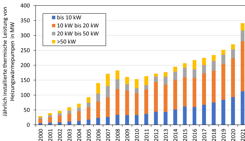
Abbildung 14 – Thermische Leistung neu installierter Heizungswärmepumpen in Österreich nach Leistungsklassen bis 2021. Quelle: ENFOS (2022)
