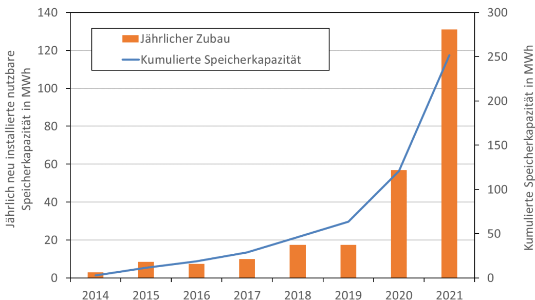
Abbildung 7 – Nutzbaere PV-Batteriespeicherkapazität in MWh bis 2021
