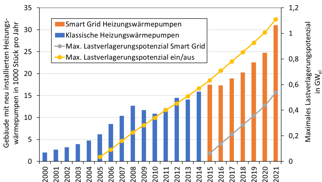
Abbildung 13 – Entwicklung des netzdienlichen Lastverlagerungspotenzials bis 2021 durch thermisch aktivierte Bauteile und Gebäude. Quelle: ENFOS (2022)
