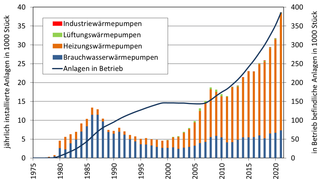
Abbildung 11 – Die Marktentwicklung der Wärmepumpen in Österreich bis 2021
