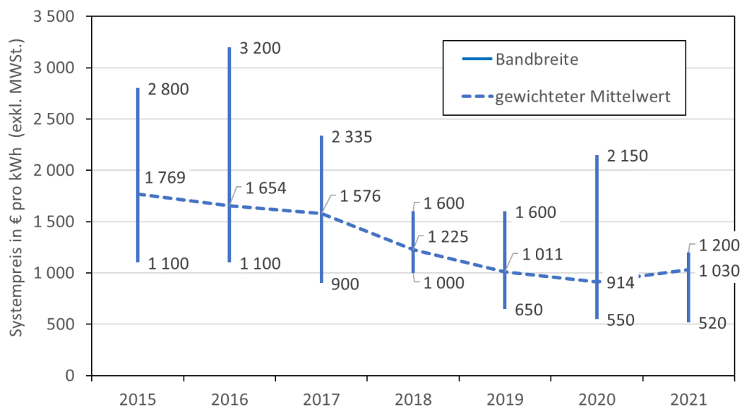
Abbildung 8 – Entwicklung der Systempreise für PV-Speichersysteme in Österreich (Mittelwert und Bandbreite) exkl. MwSt. pro kWh nutzbare Speicherkapazität
